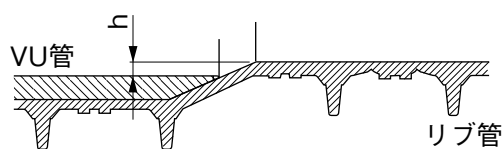
A部詳細図
