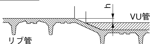
A部詳細図
