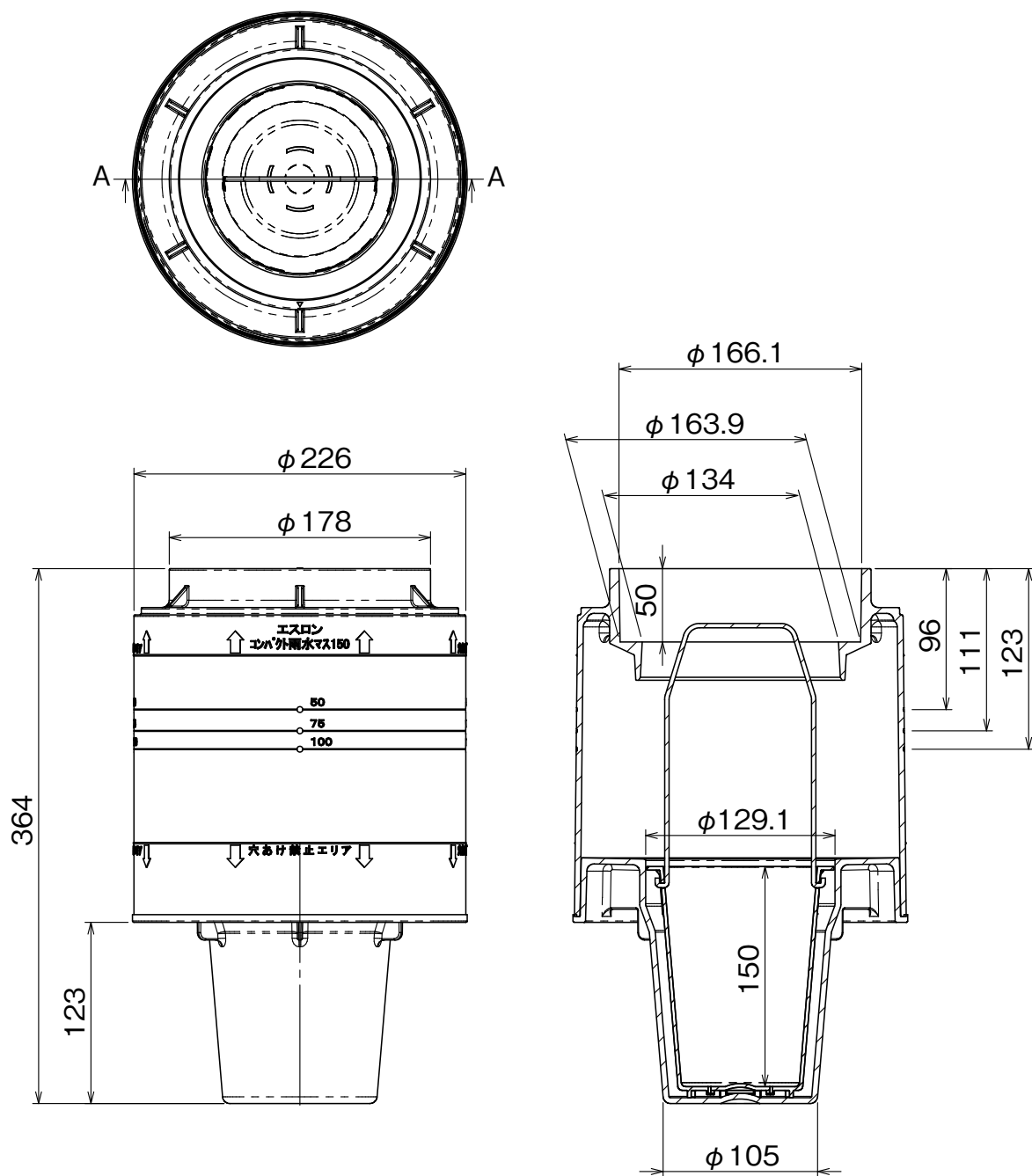
断面図 A-A
